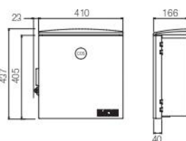
TOKERUMO制御盤外形図
